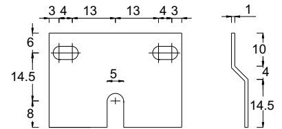
Unit:mm Material:1mm steel No :MT01
